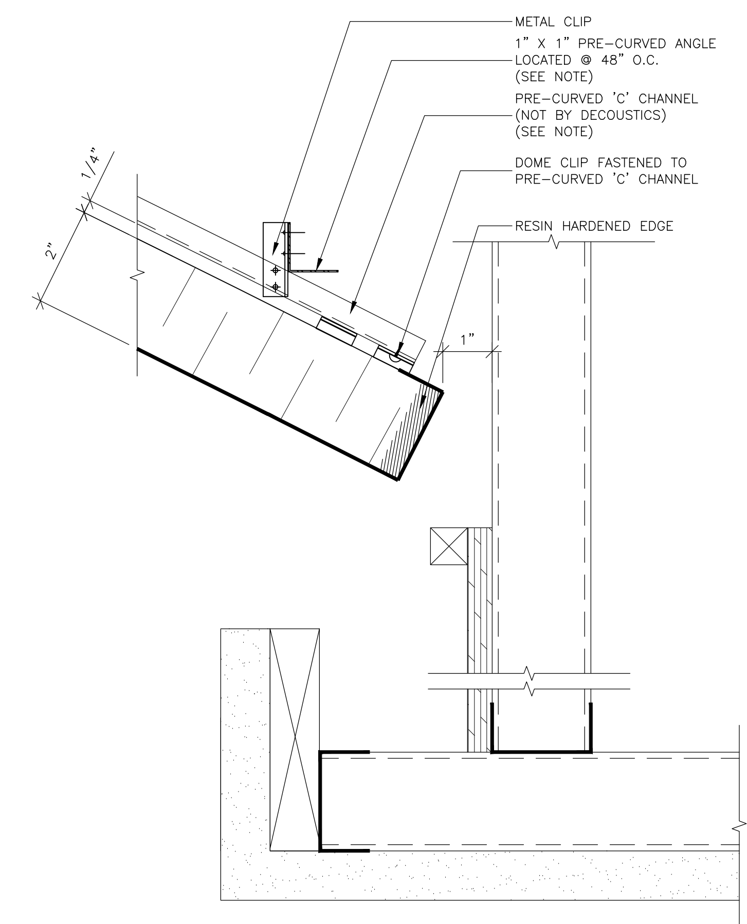
5 PERIMETER DETAIL SCALE: 6" = 1'-0"
