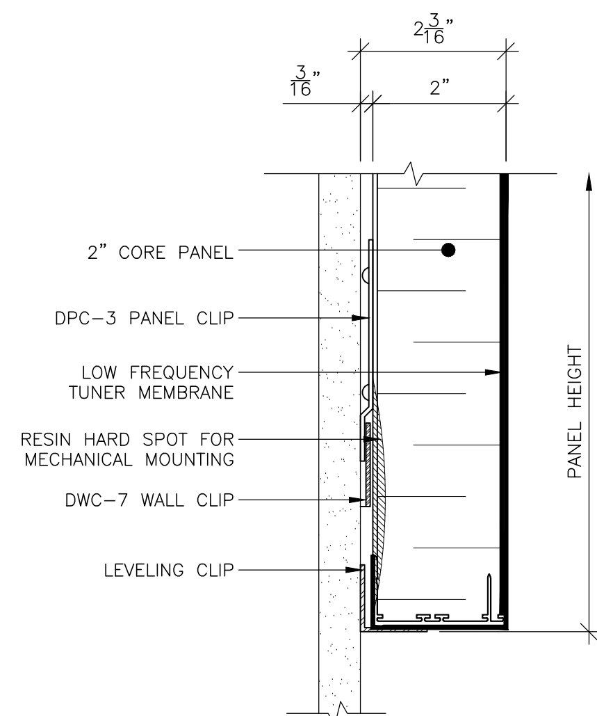
6 PANEL BASE @ WALL SCALE: 6" = 1'-0" REF: D1
