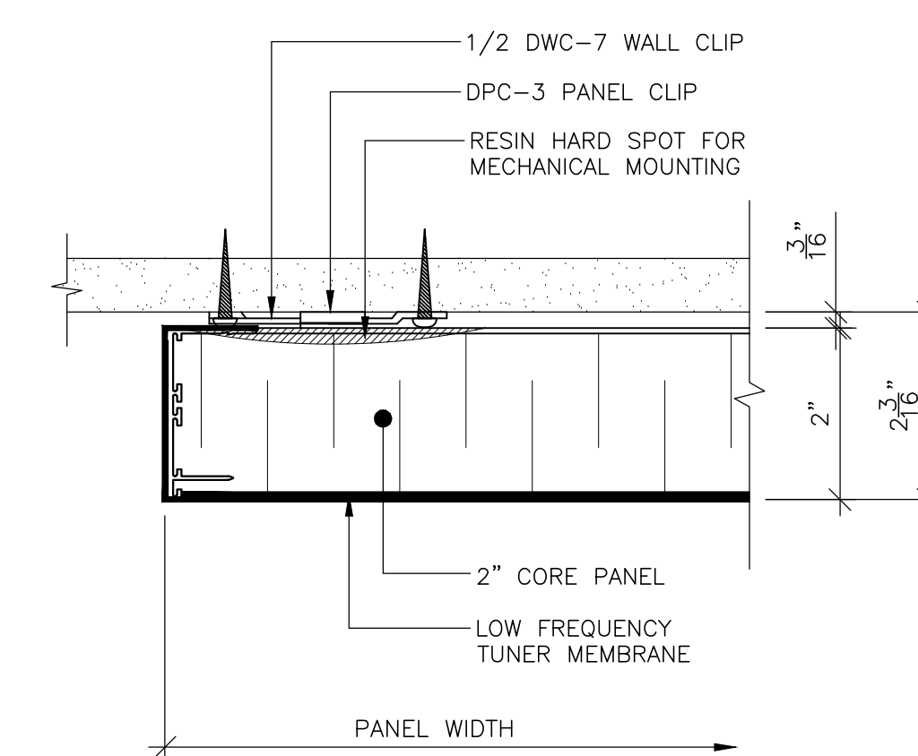
6 PANEL BASE @ WALL SCALE: 6" = 1'-0" REF: D1
