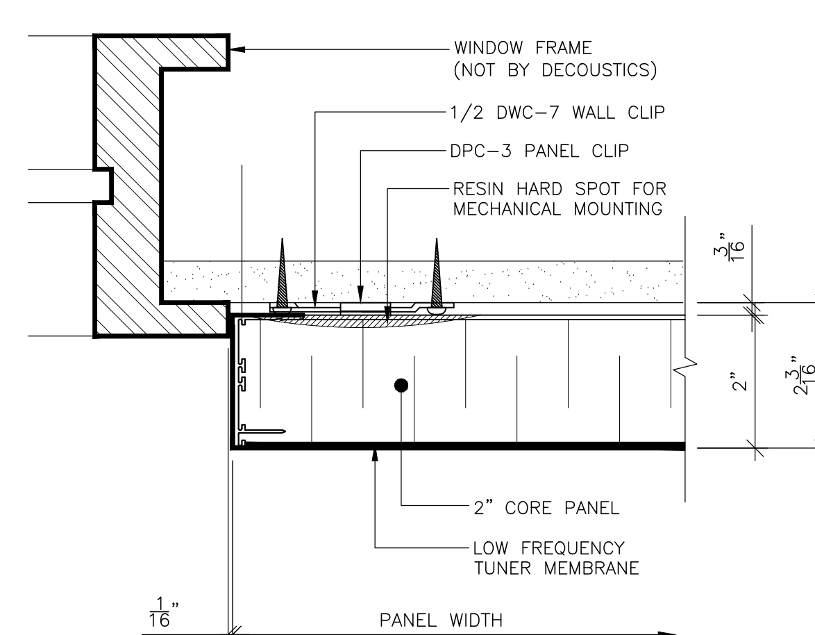
11 PANEL END @ FRAME SCALE: 6" = 1'-0" REF: D1
