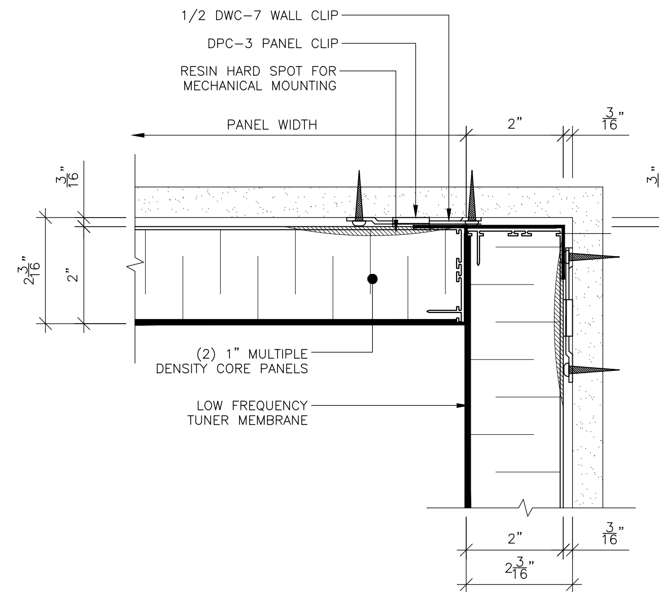
7 PANEL END @ CORNER SCALE: 6" = 1'-0" REF: D1
