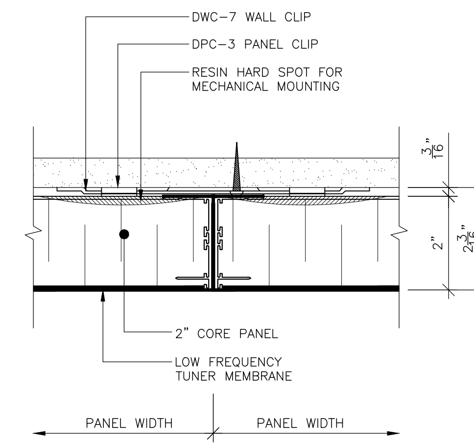
4 VERT. BUTT JOINT DET. SCALE: 6" = 1'-0" REF: D1
