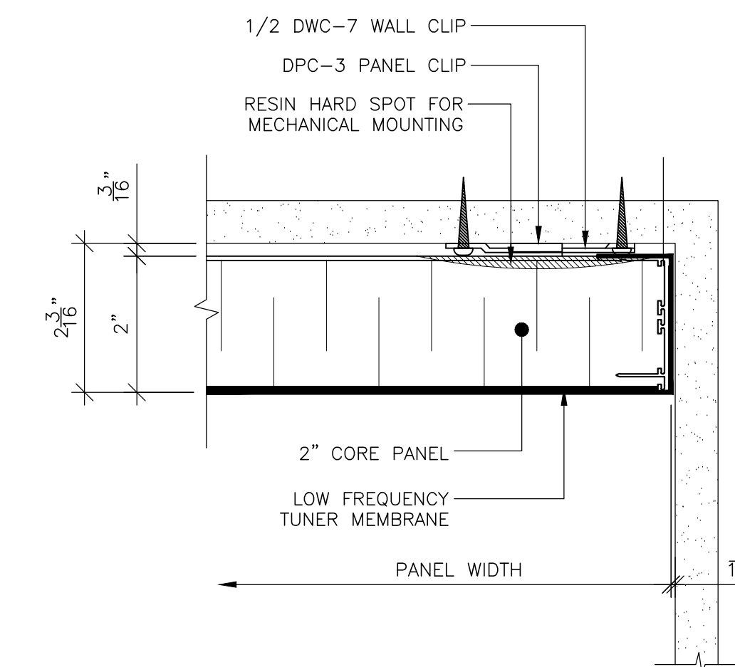
8 PANEL END @ WALL SCALE: 6" = 1'-0" REF: D1
