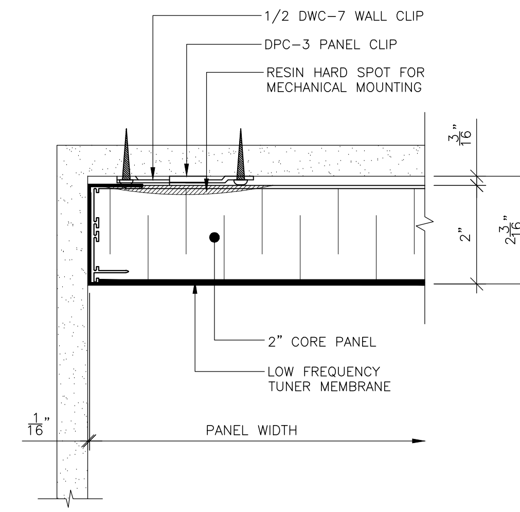
3 PANEL END @ WALL SCALE: 6" = 1'-0" REF: D1
