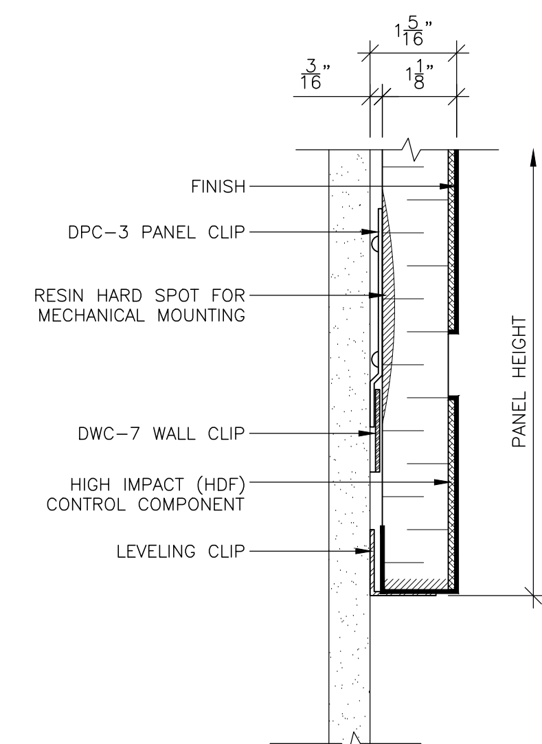
6 PANEL BASE @ WALL SCALE: 6" = 1'-0" REF: D1
