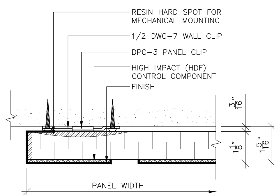
10 PANEL END @ WALL SCALE: 6" = 1'-0" REF: D1
