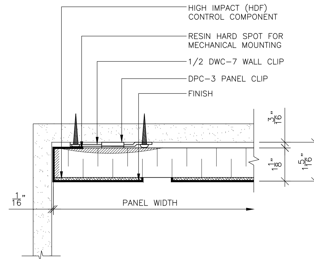
3 PANEL END @ WALL SCALE: 6" = 1'-0" REF: D1
