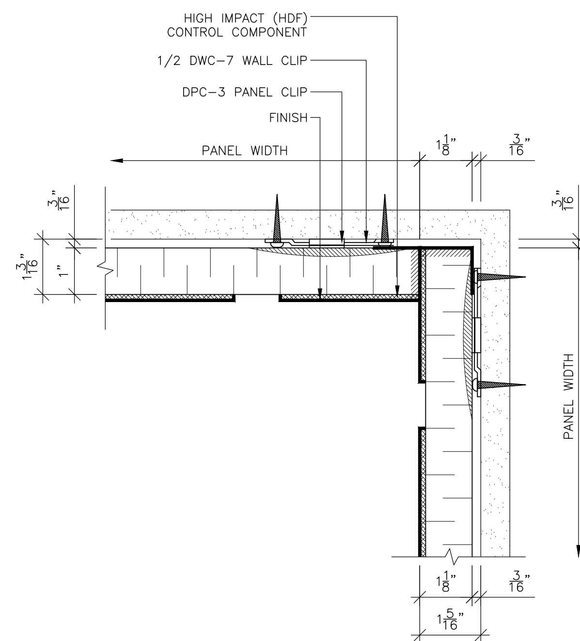
7 PANEL END @ CORNER SCALE: 6" = 1'-0" REF: D1
