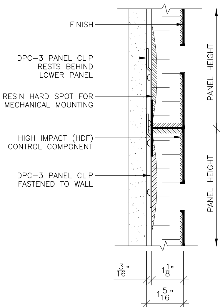
9 HORIZ. BUTT JOINT DET. SCALE: 6" = 1'-0" REF: D1
