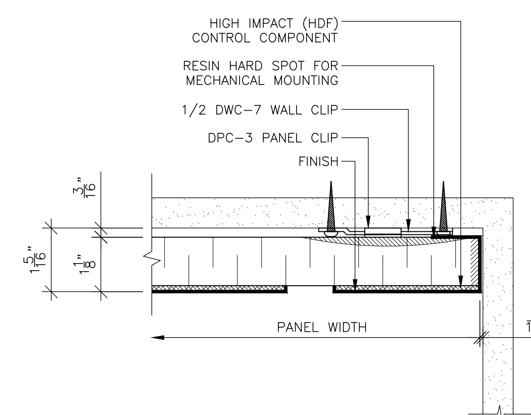
8 PANEL END @ WALL SCALE: 6" = 1'-0" REF: D1
