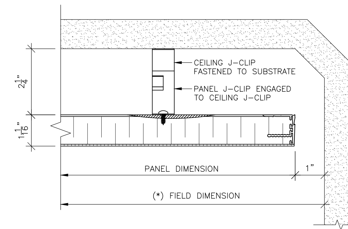
6 PERIMETER PANEL DETAIL D1 SCALE: 6" = 1'-0"
