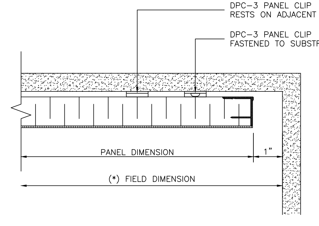
8 PANEL PERIMETER DETAIL D1 SCALE: 1/2"=1"
