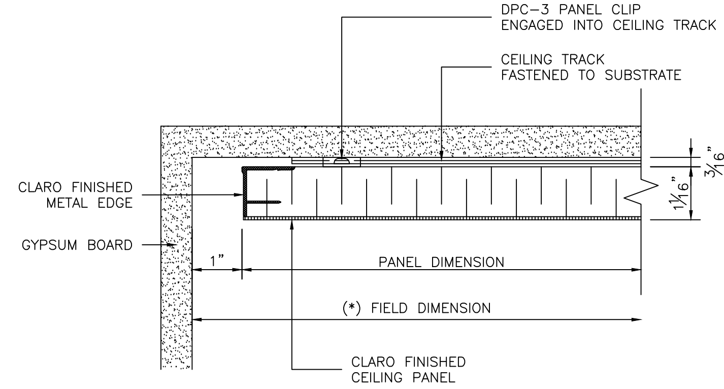
5 PANEL PERIMETER DETAIL D1 SCALE: 1/2"=1"
