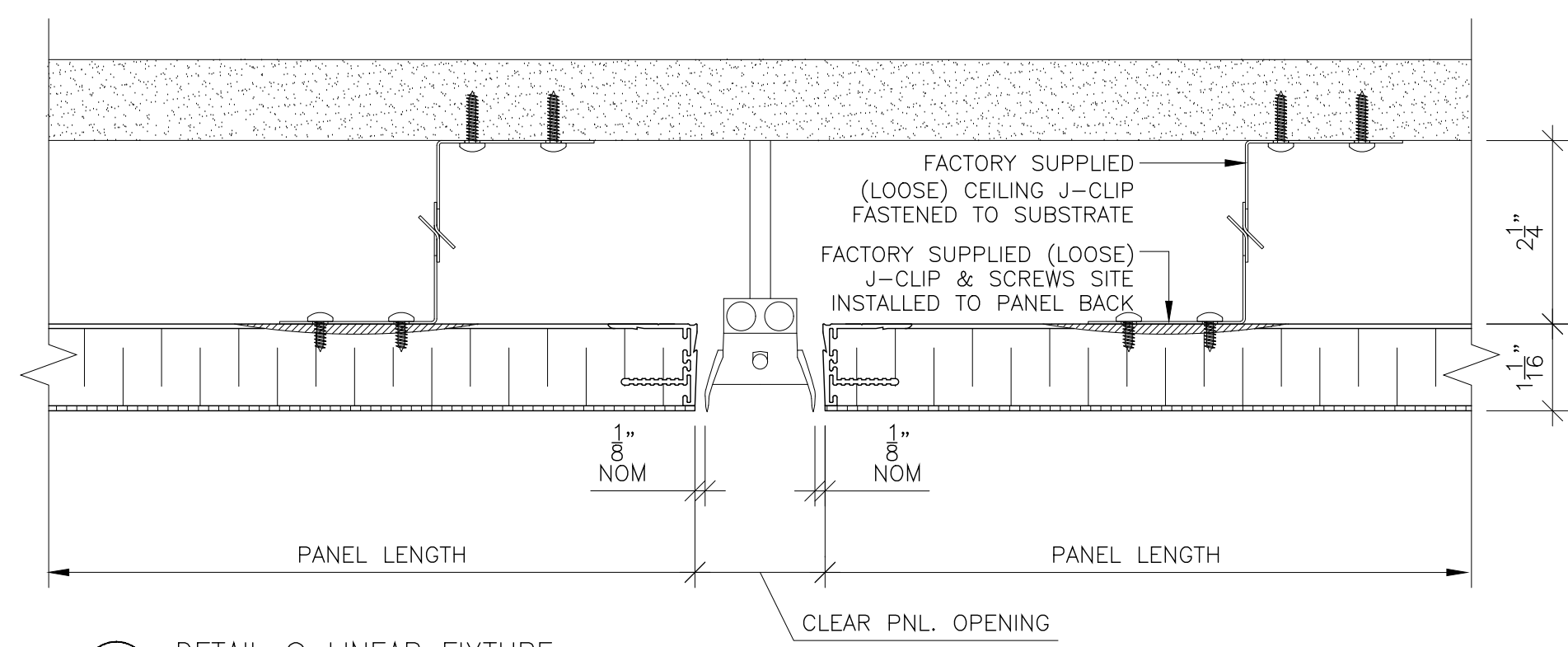
7 DETAIL @ LINEAR FIXTURE SCALE: 6" = 1'-0"
