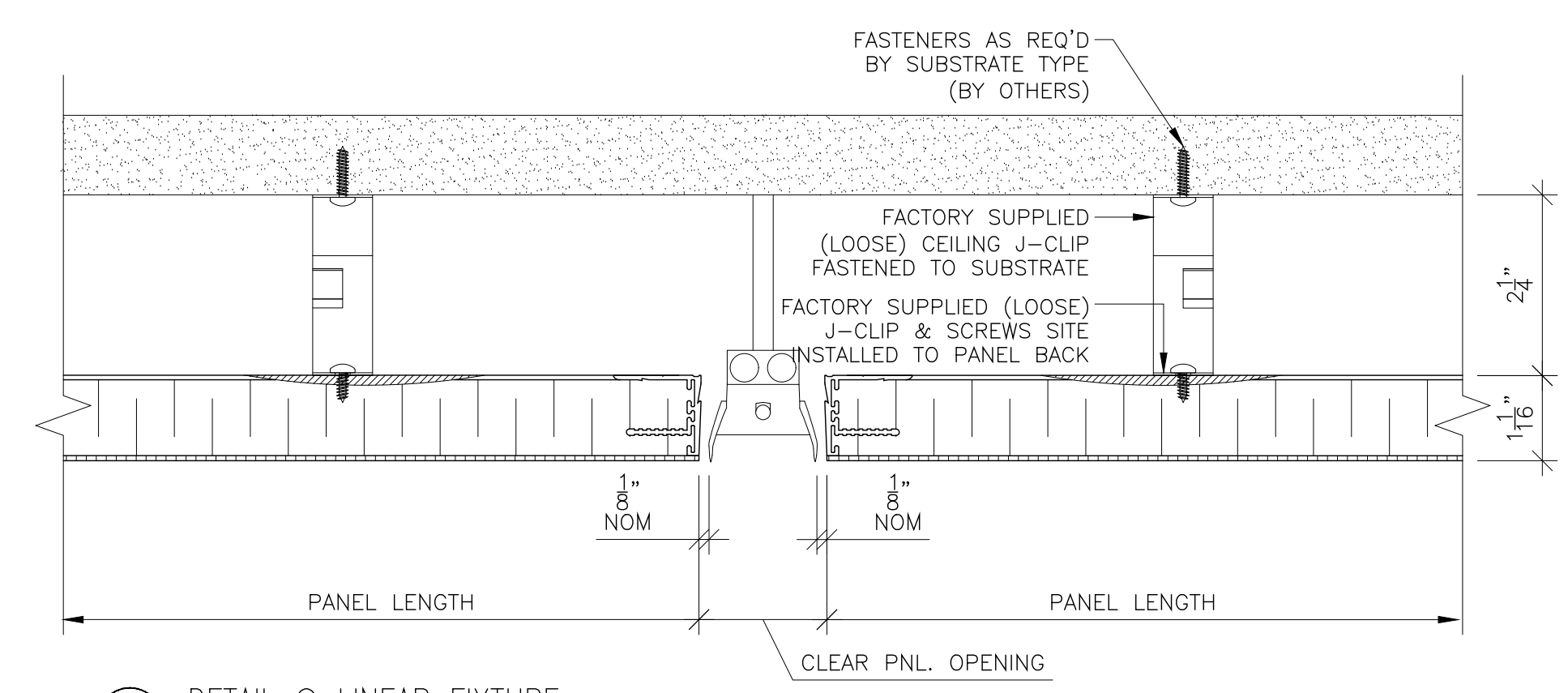
8 DETAIL @ LINEAR FIXTURE SCALE: 6" = 1'-0"
