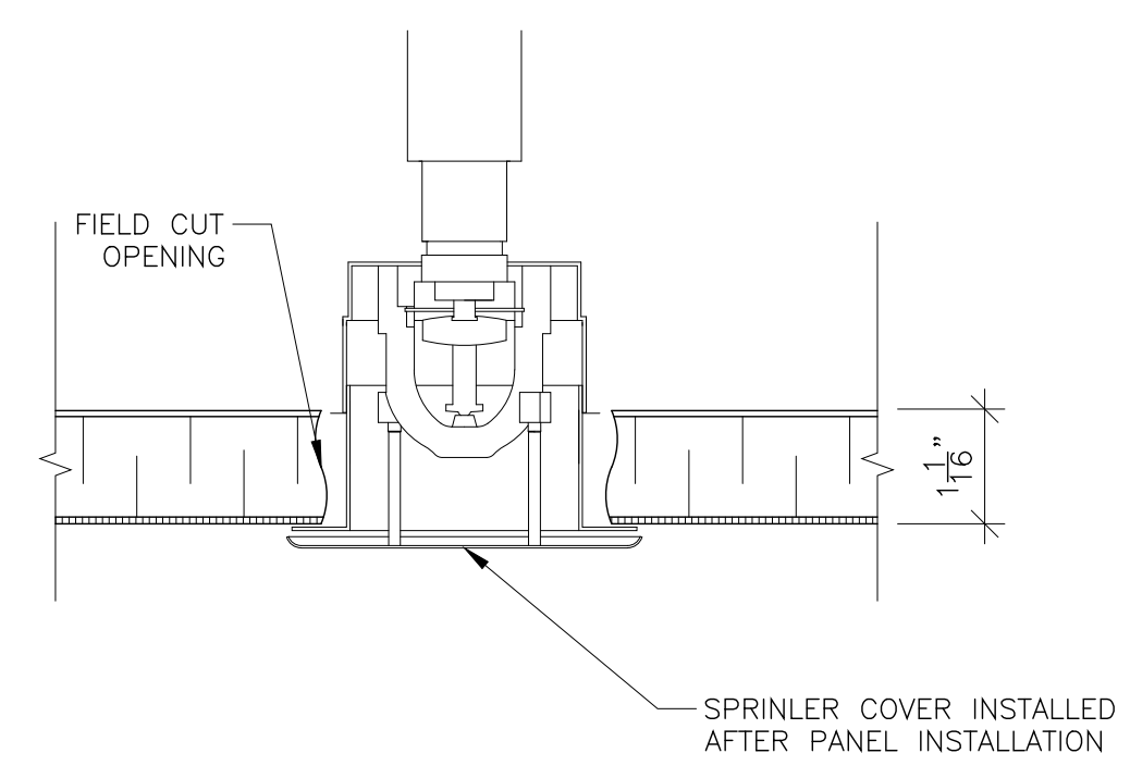
9 DETAIL @ SPRINKLER SCALE: 6" = 1'-0"
