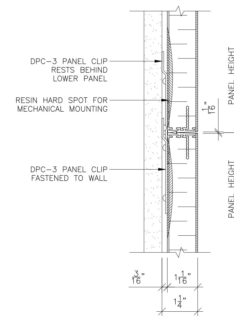
8 HORIZ. BUTT JOINT DET. SCALE: 6" = 1'-0" REF:
